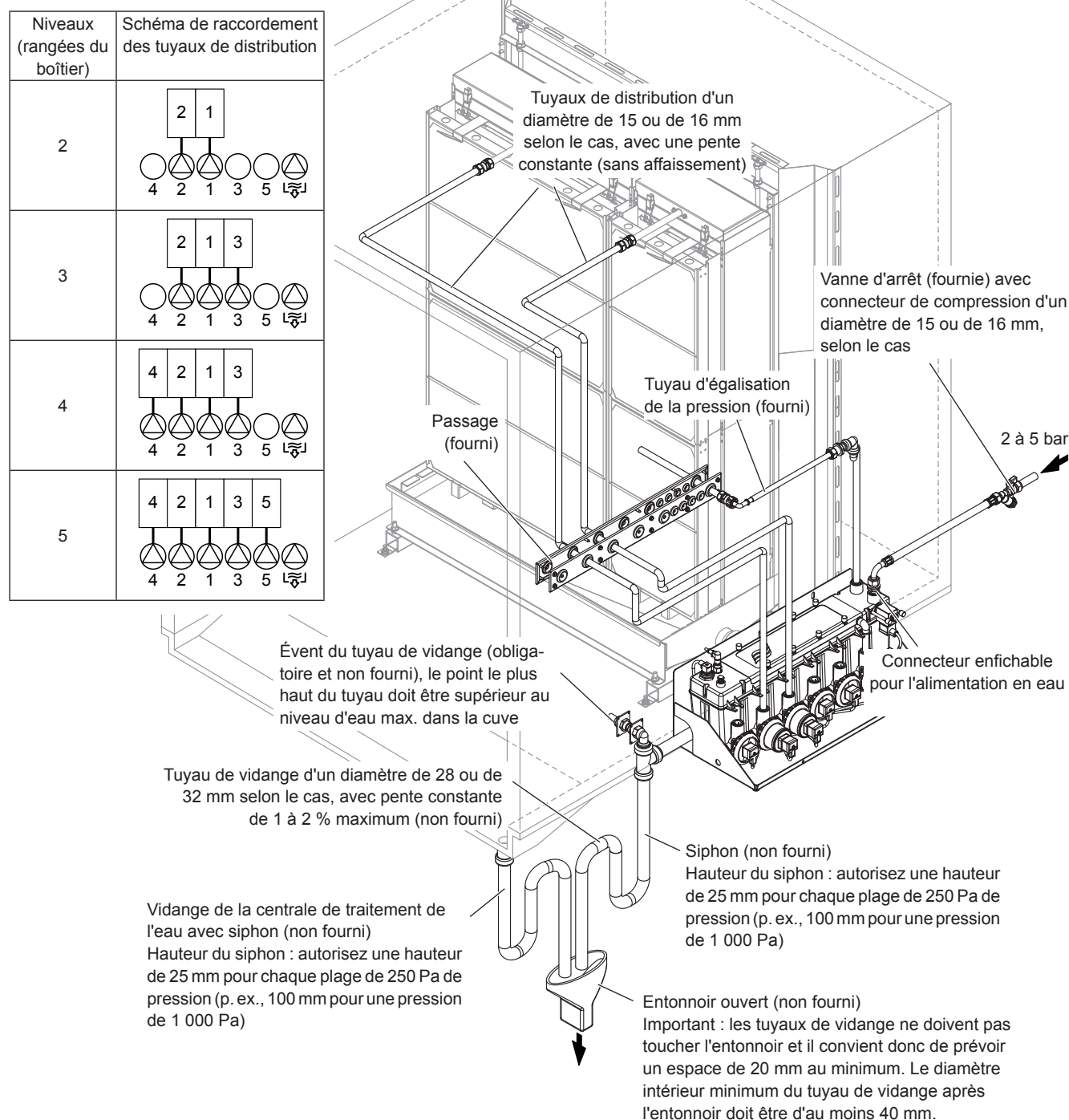
Fig. 32 : Installation du circuit d'eau (installation externe)
