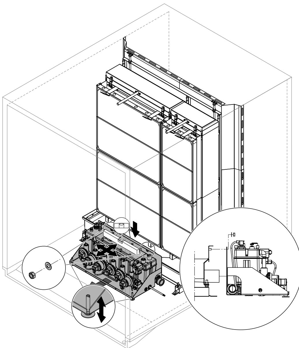
Fig. 19 : Montage du module hydraulique (installation interne)
