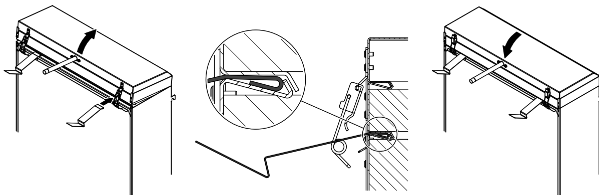
Fig. 16 : Installer les supports du séparateur de gouttelettes
