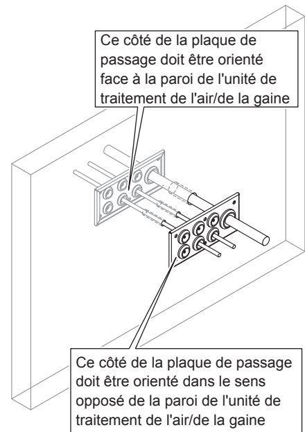
Fig. 28 : Montage de la plaque de passage (installation interne)
