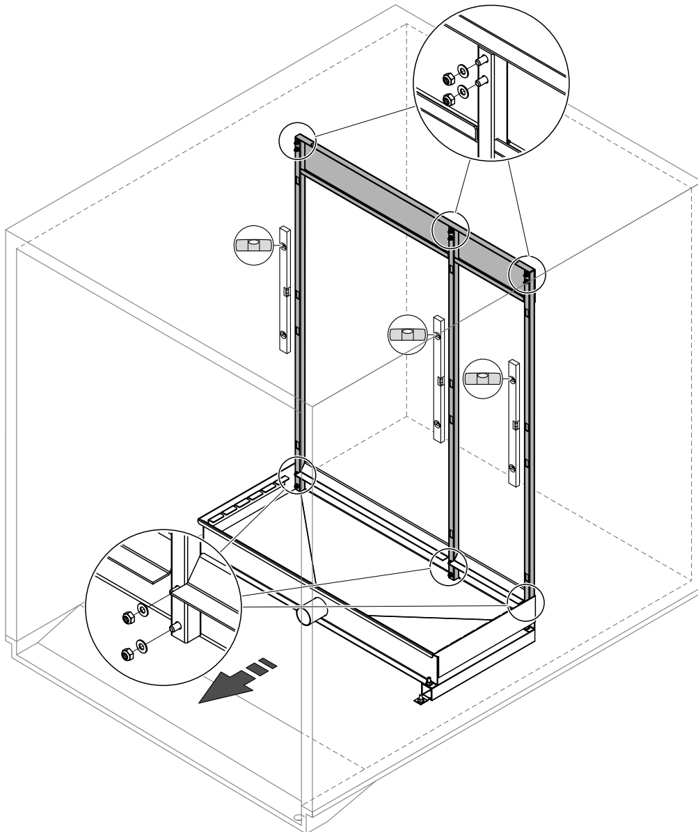
Fig. 7 : Fixation du cadre à la cuve
