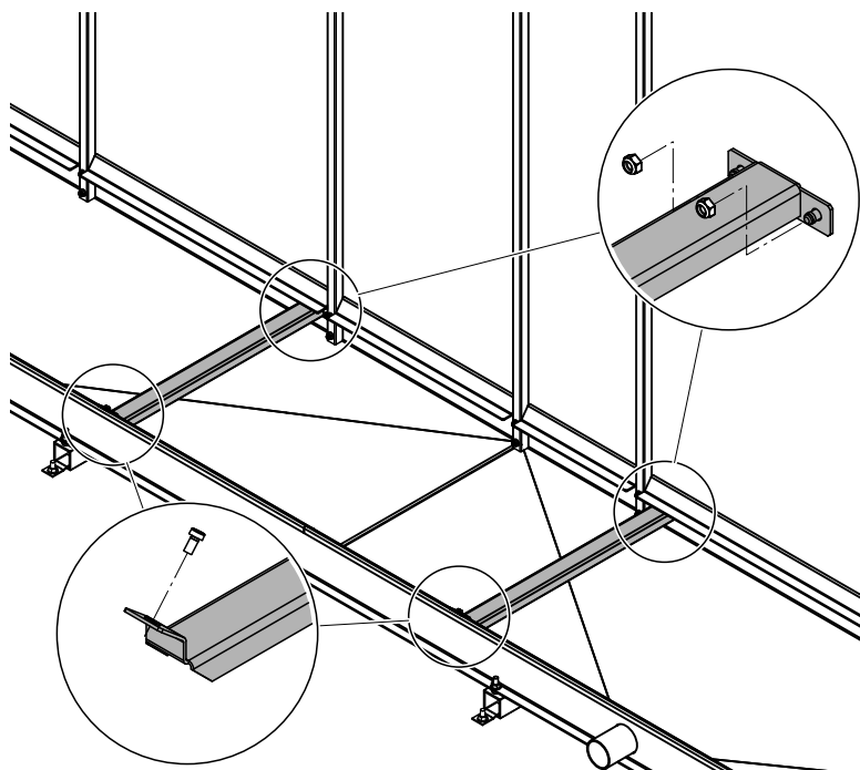
Fig. 10 : Montage du/des support(s) de la barre transversale
