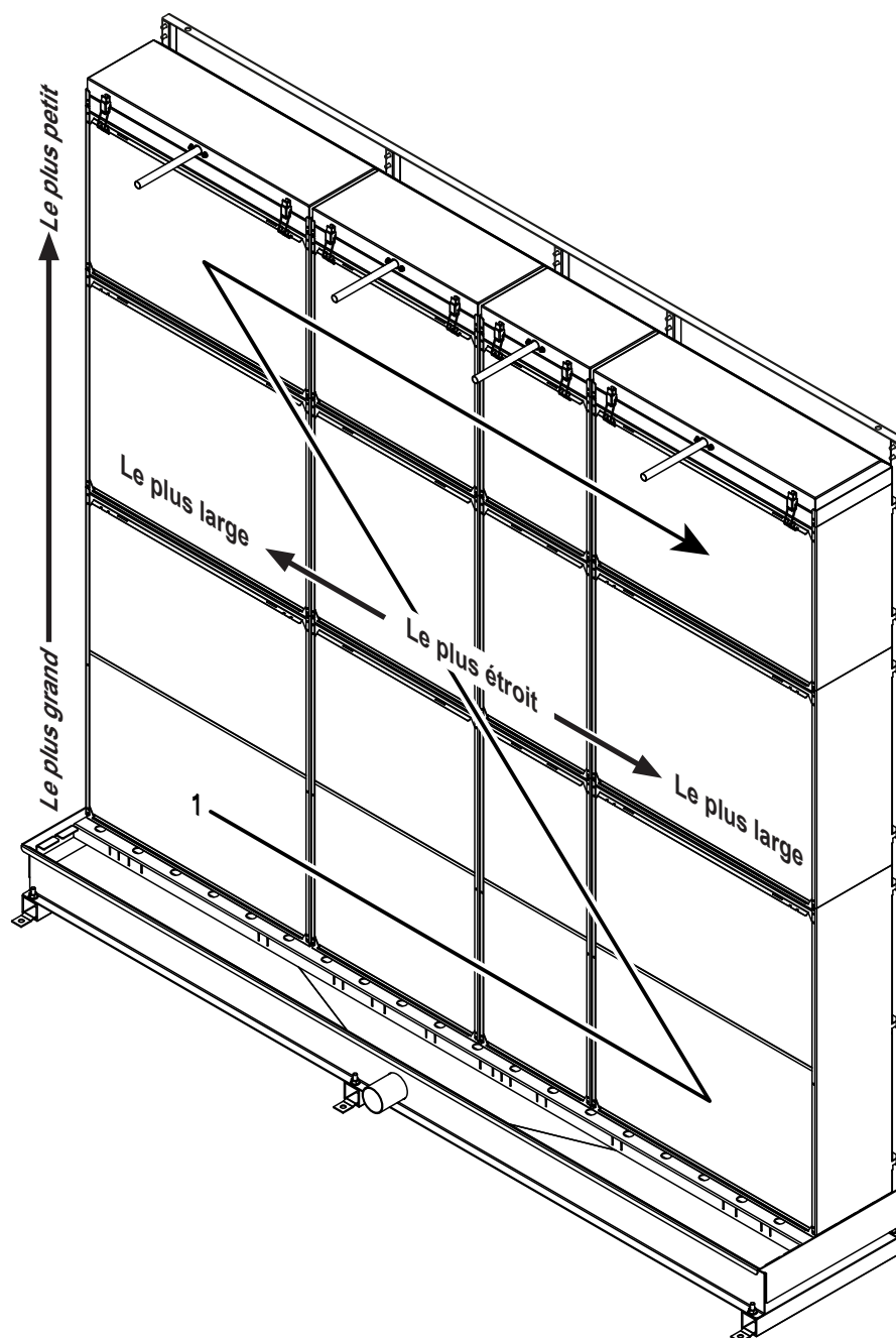
Fig. 15 : Ordre de montage et positionnement des cassettes d'évaporation
