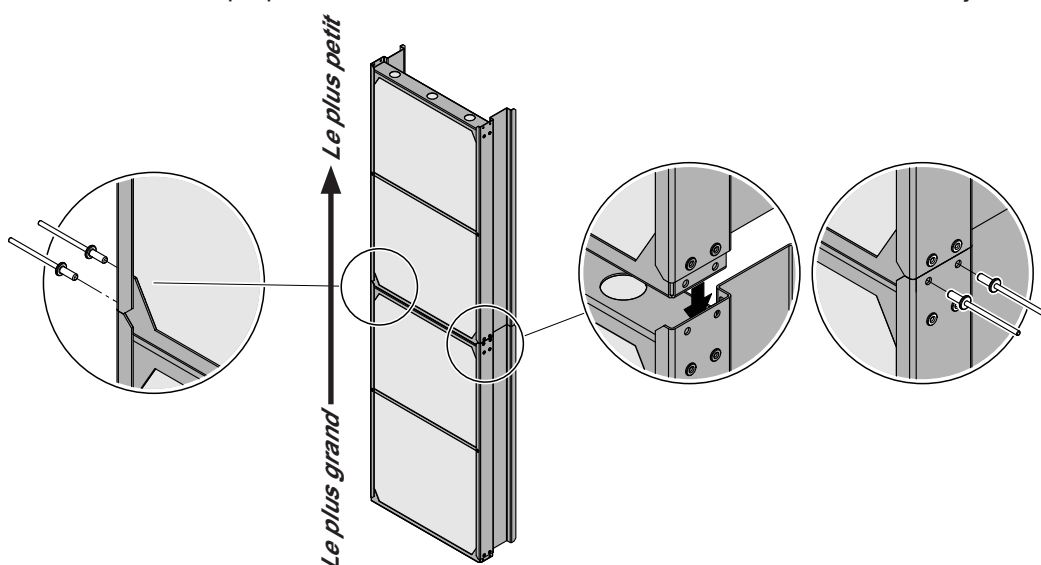
Fig. 17 : Rivetage des bancs des cassettes de séparateur de gouttelettes ensemble
