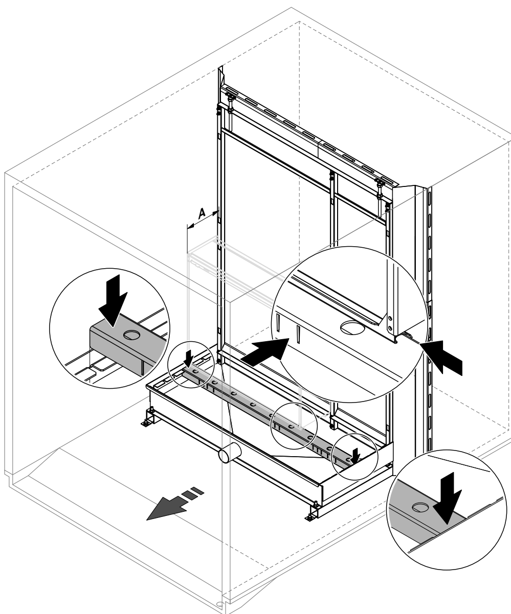
Fig. 11 : Montage de la barre transversale
