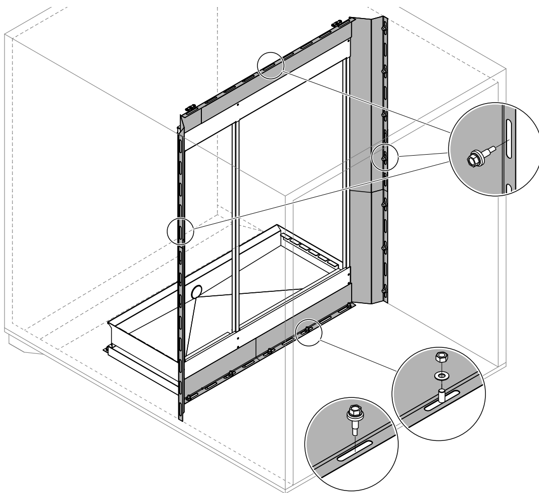
Fig. 9 : Montage des plaques d'obturation Condair (disponibles en option) sur le côté de l'admission d'air
