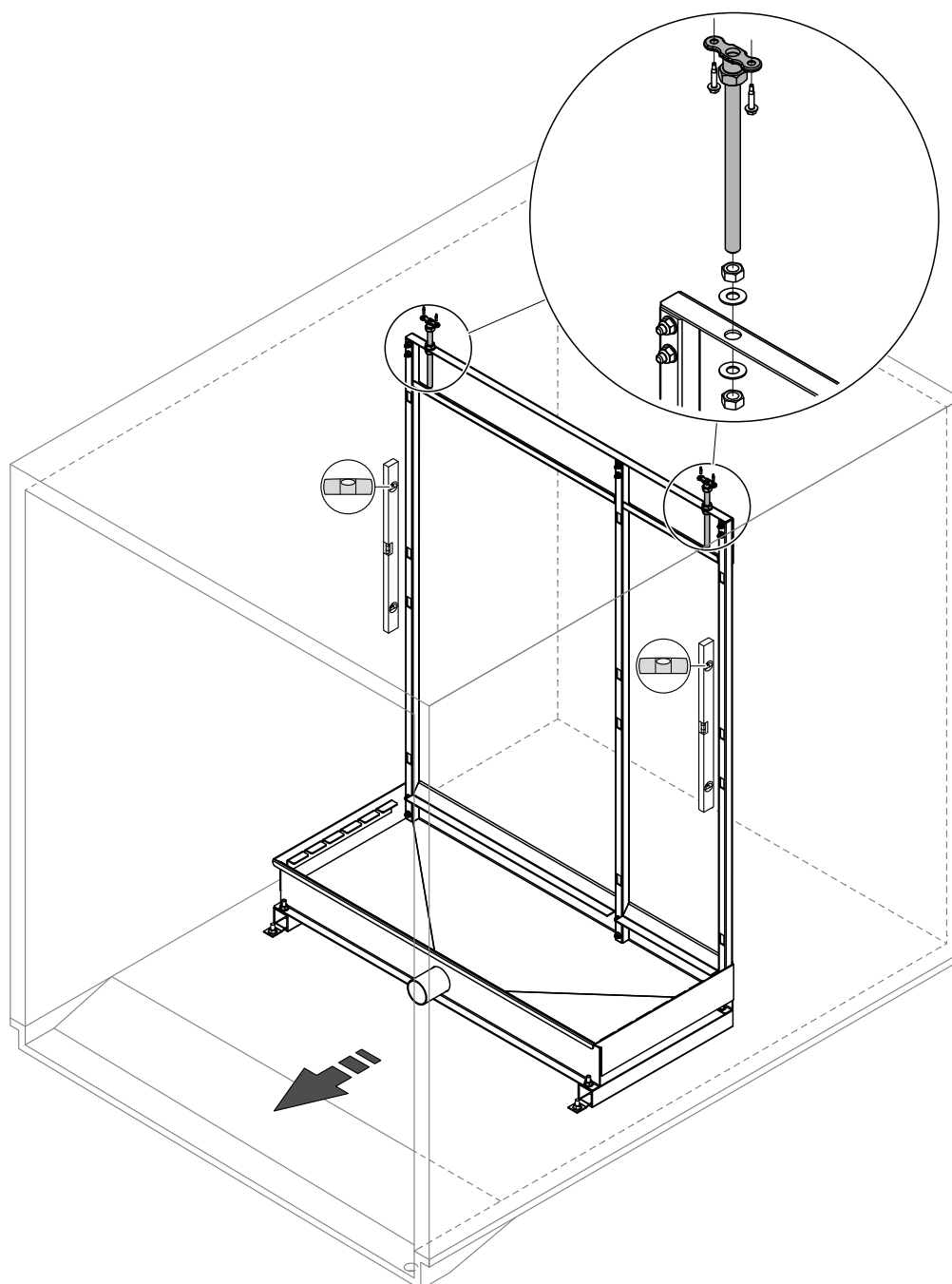
Fig. 8 : Fixation de la barre transversale à la paroi supérieure de l'unité de traitement de l'air/de la gaine d'aération
