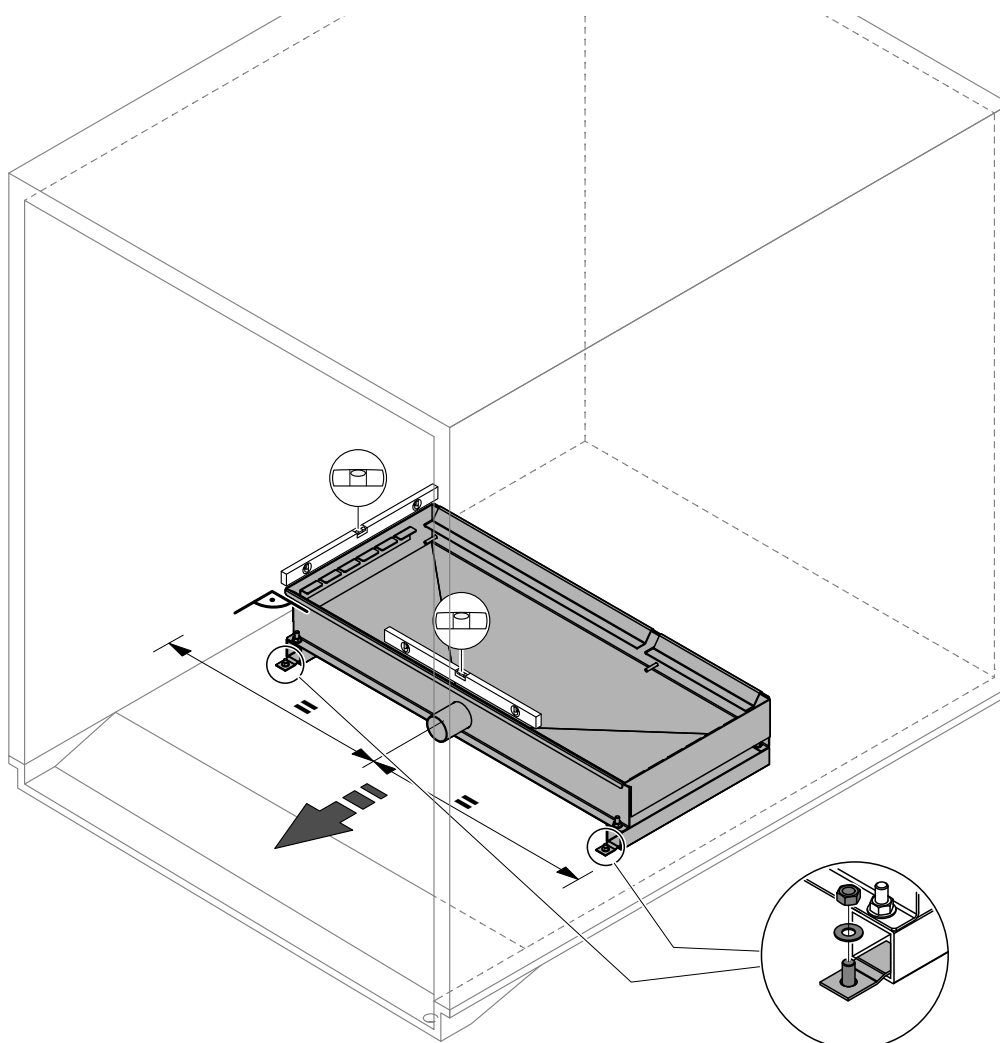
Fig. 6 : Montage de la cuve
