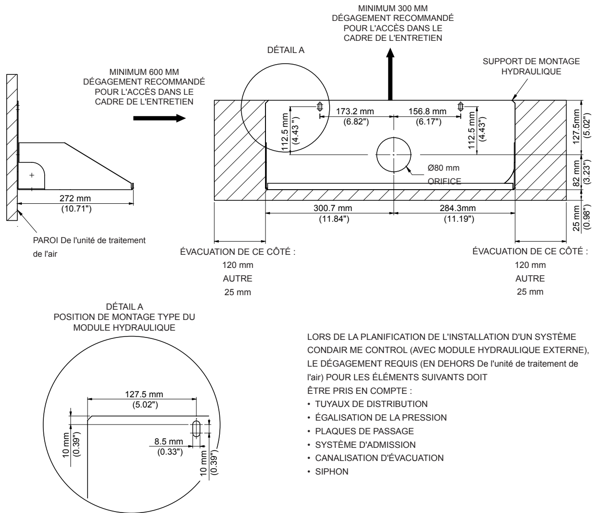
Fig. 20 : Espaces à respecter lors du montage externe du module hydraulique
