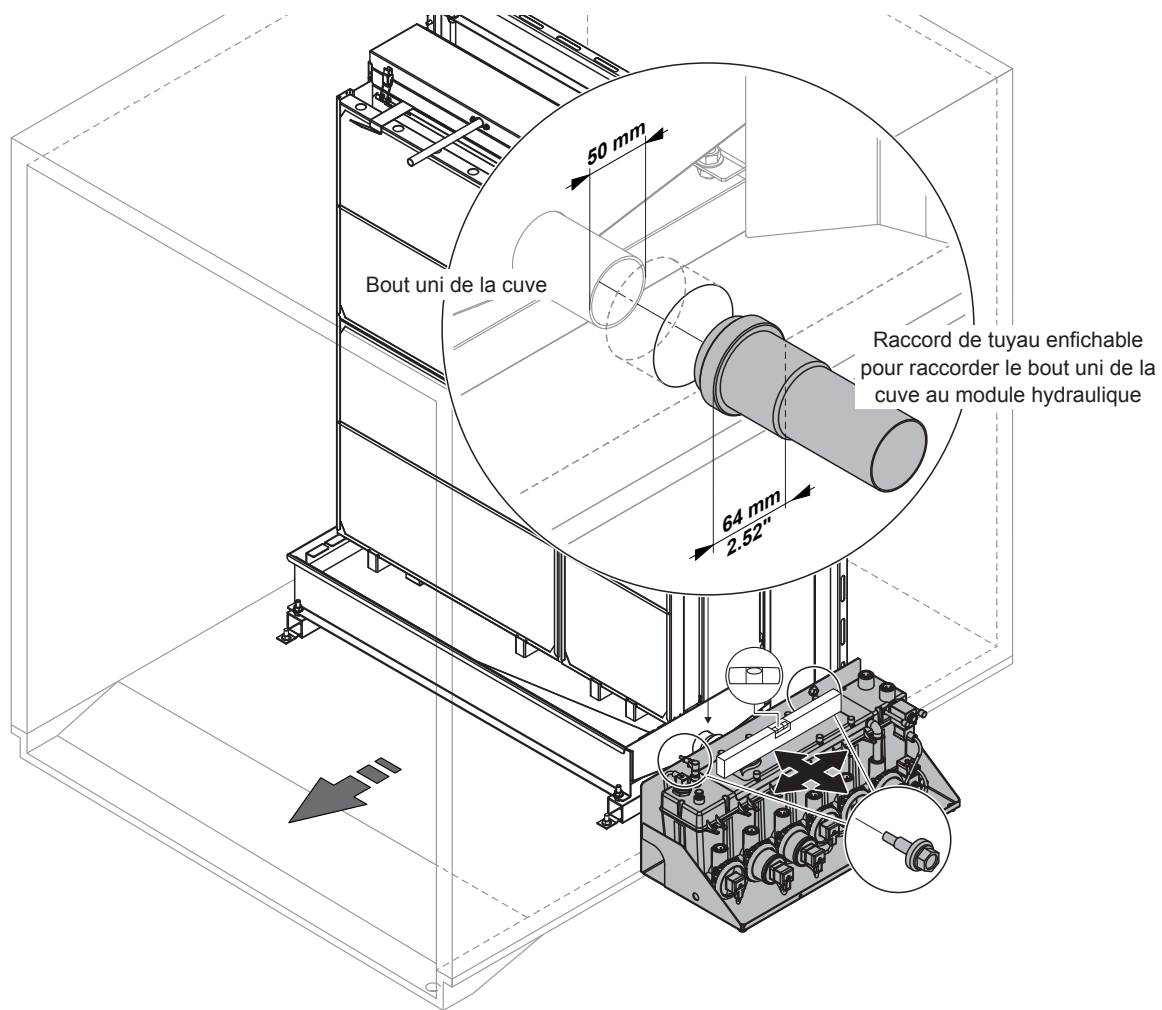
Fig. 22 : Montage du module hydraulique (installation externe, cuve de vidange latérale)
