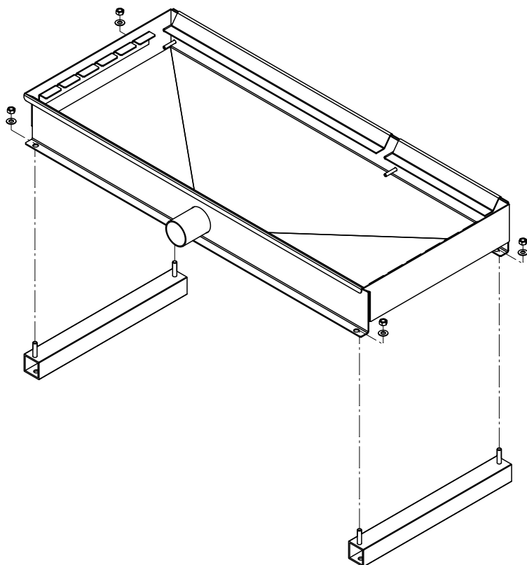
Fig. 5 : Montage des supports sur la cuve
