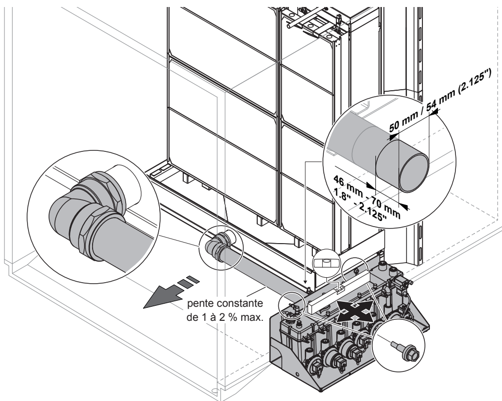
Fig. 21 : Montage du module hydraulique (installation externe, cuve de vidange centrale)
