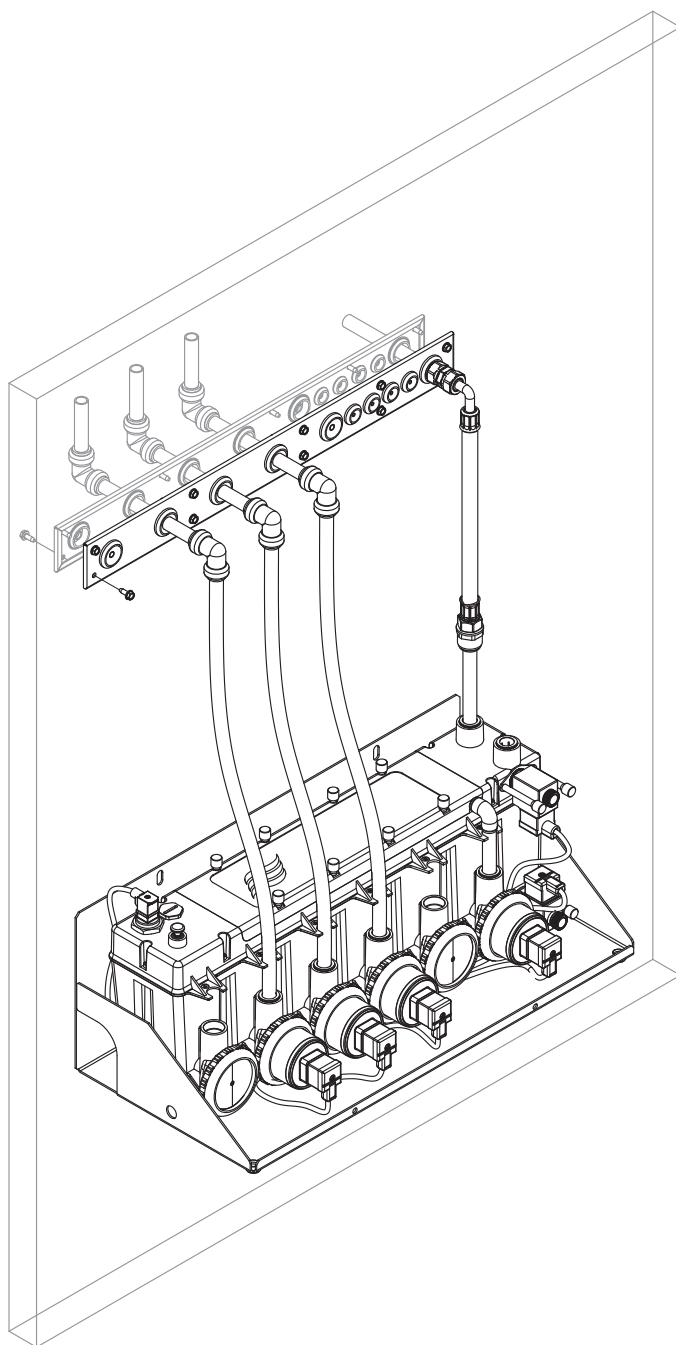
Fig. 29 : Fixation de la plaque de passage sur la paroi du conduit (installation externe)
