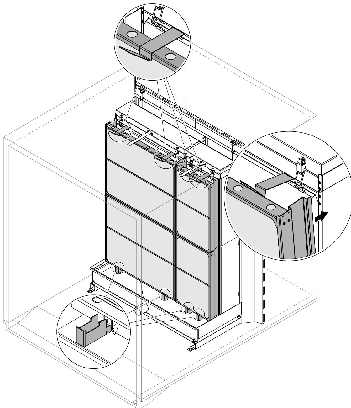
Fig. 18 : Montage des bancs du séparateur de gouttelettes
