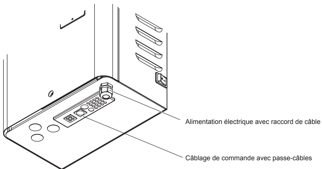
Fig. 35 : Passe-câbles de l'unité de commande
