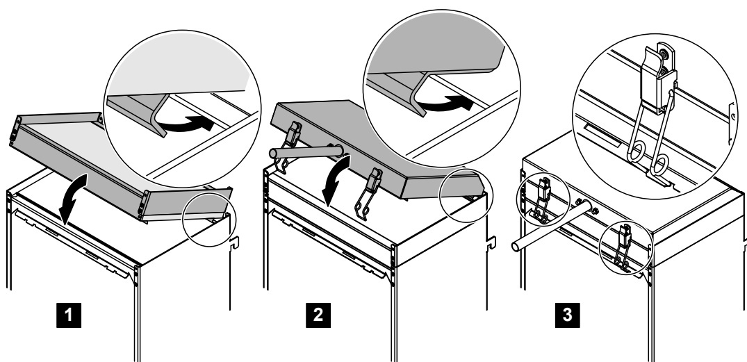
Fig. 12 : Montage de la tête de distribution sur des cassettes d'évaporation en fibre de verre
