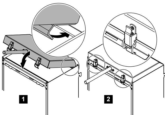
Fig. 13 : Montage de la tête de distribution sur des cassettes d'évaporation en polyester
