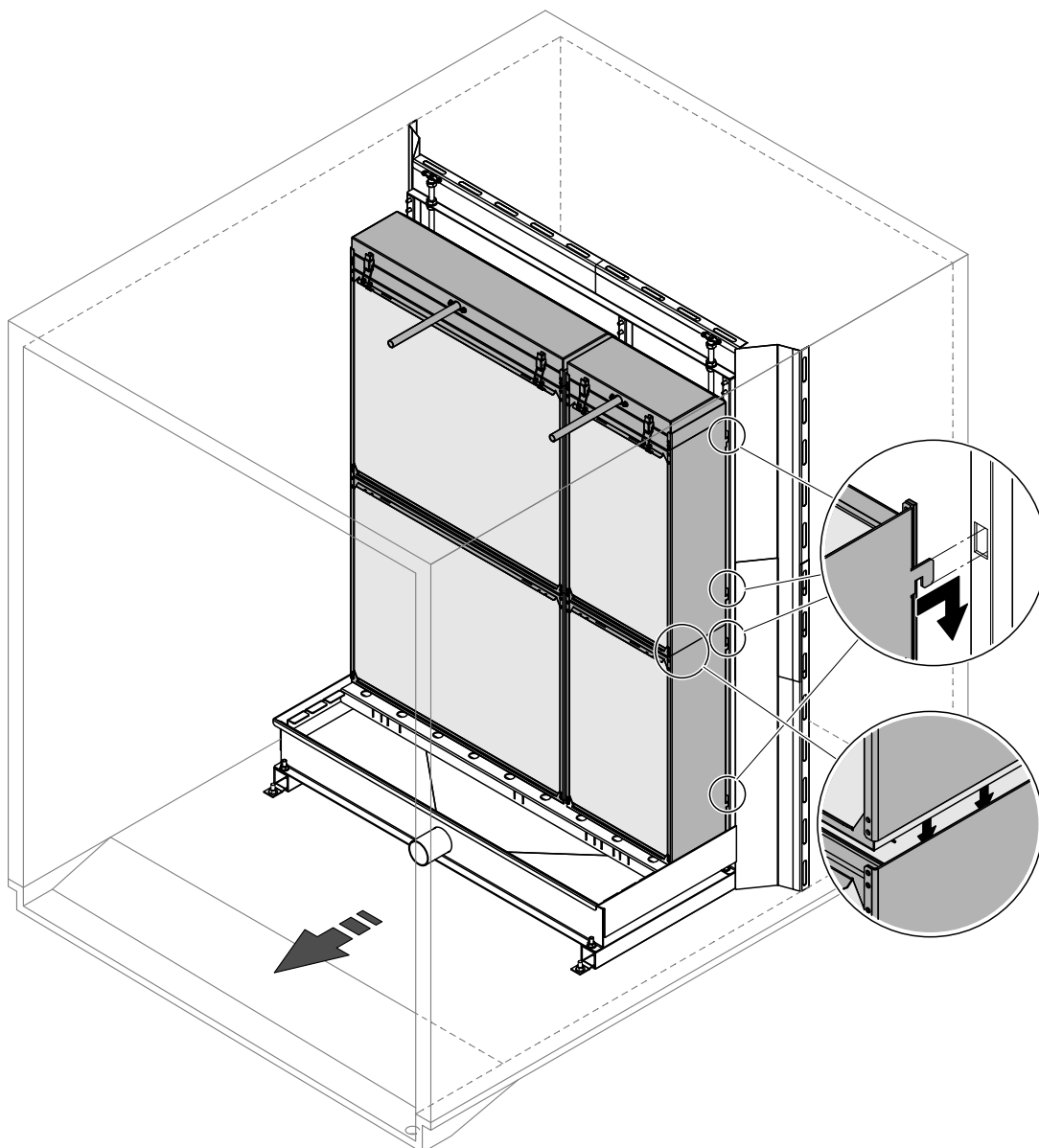
Fig. 14 : Montage des cassettes d'évaporation
