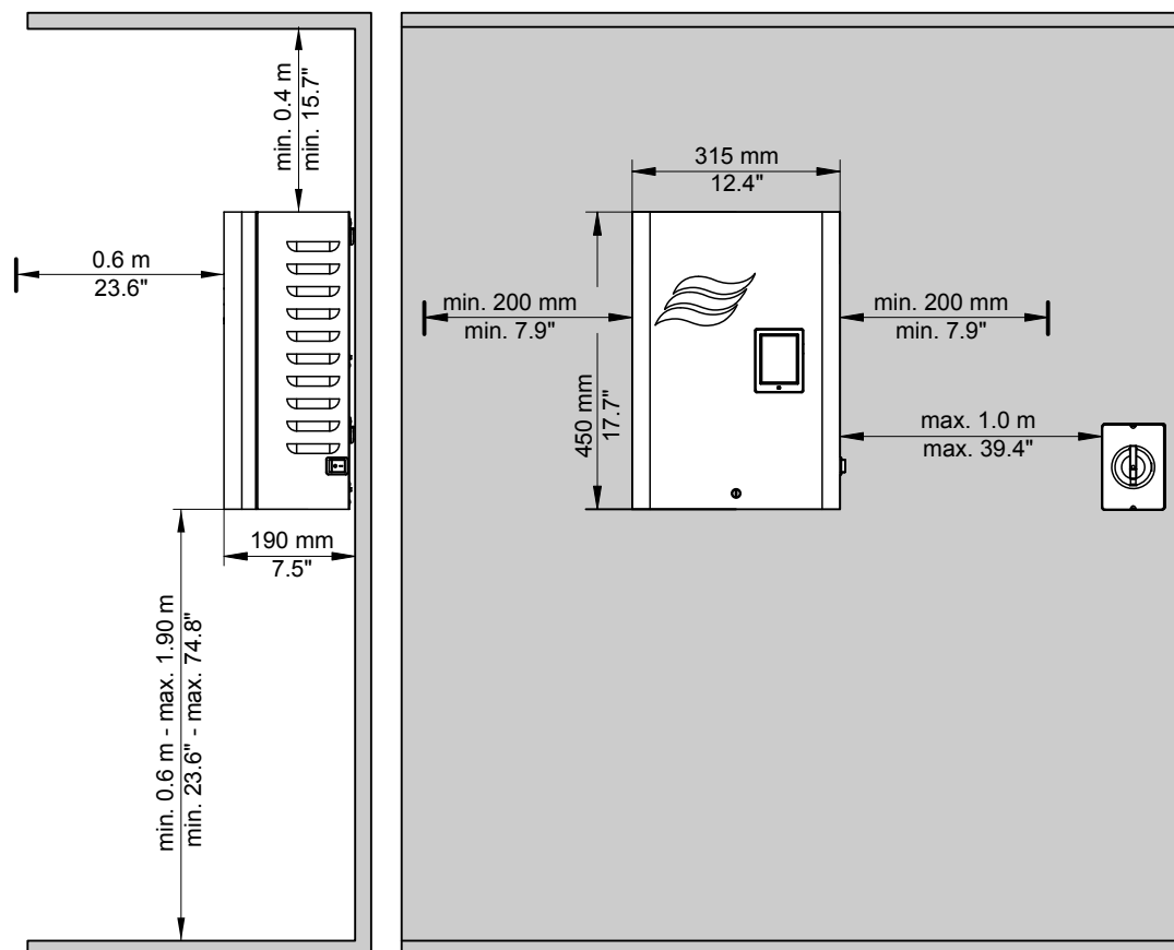
Fig. 33 : Recommandations en matière d'accessibilité de l'unité de commande
