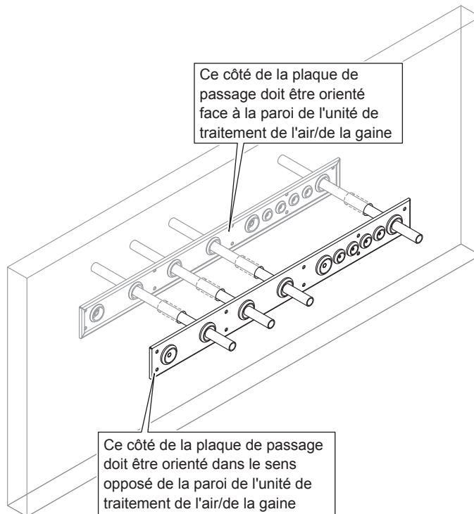
Fig. 27 : Montage de la plaque de passage (installation externe)
