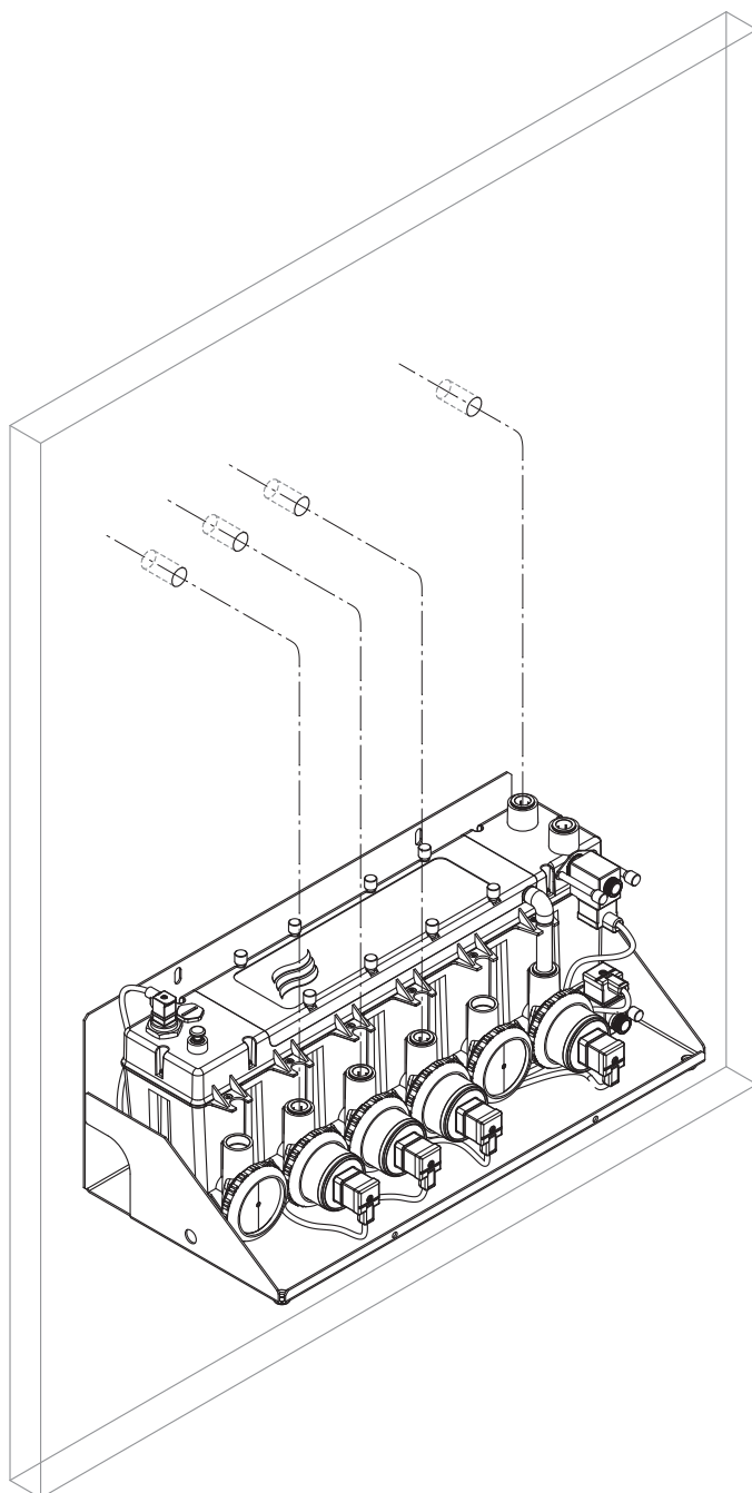
Fig. 25 : Perçage des trous de passage (installation externe)
