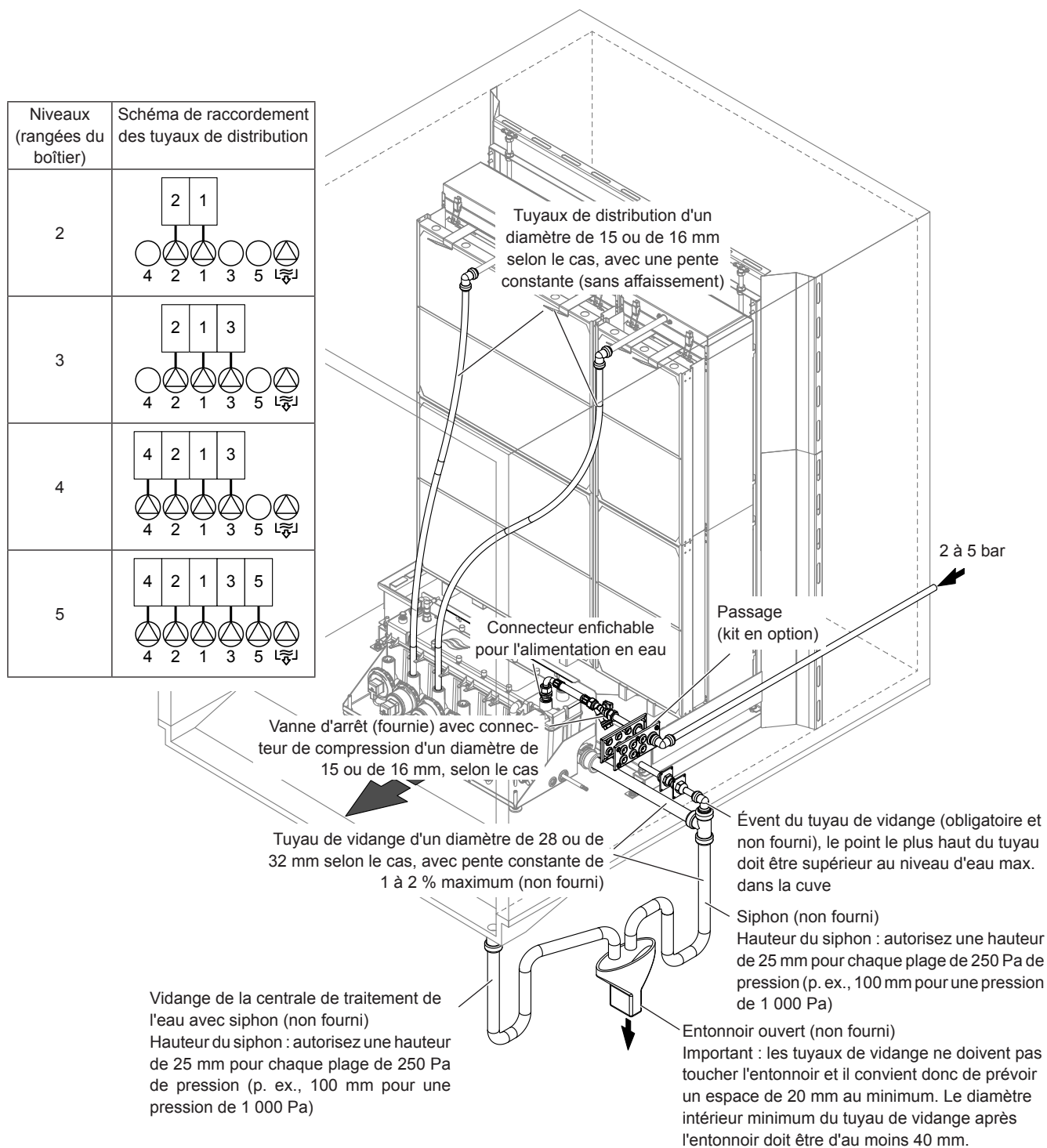
Fig. 31 : Installation du circuit d'eau (installation interne)
