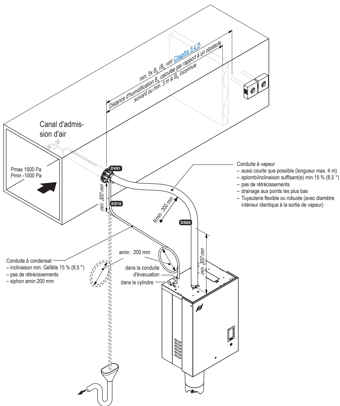
Fig. 15: Aperçu de l'installation à vapeur d'humidification d'air de gaine
